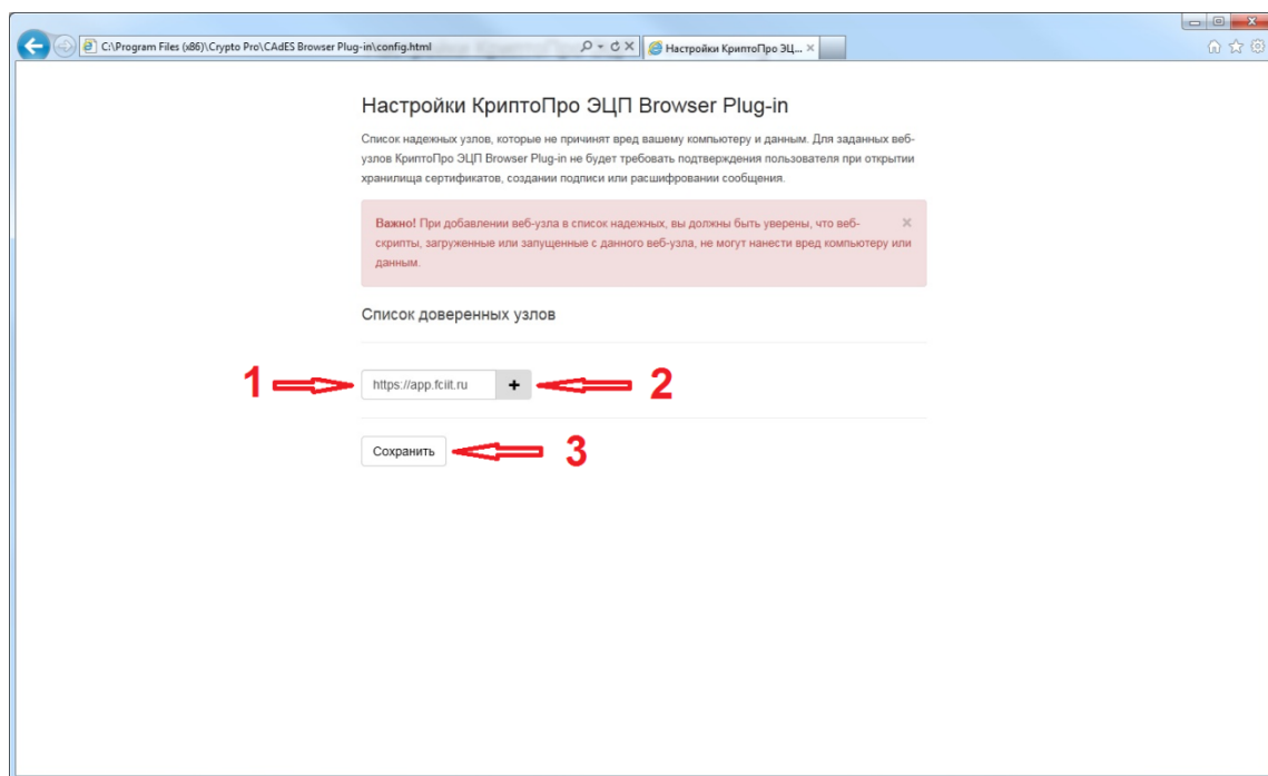
Рис 1. Настройки ЭЦП Browser Plug-in
