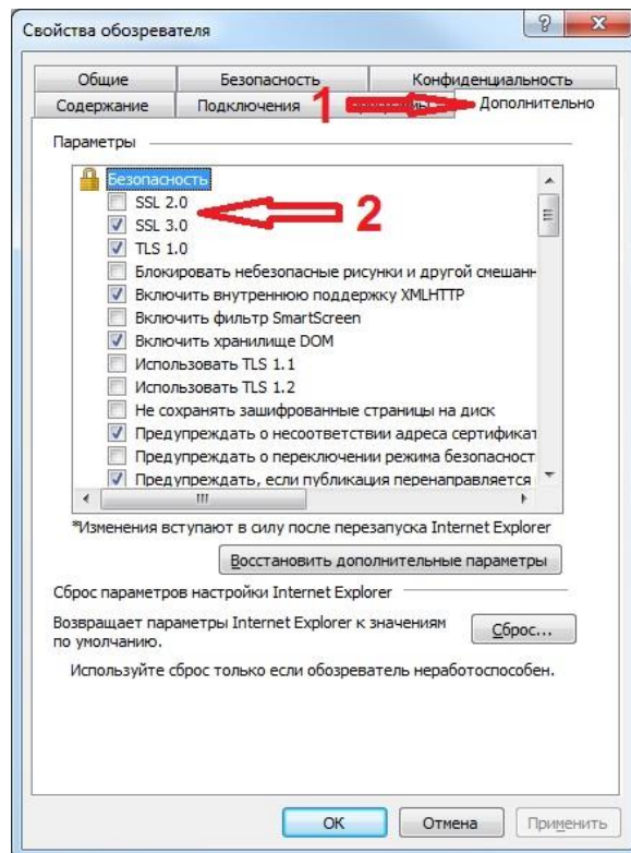
Рис 3. Включение протокола SSL
